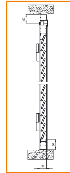
Mod. MONTECARLO con telaio su 3 lati
